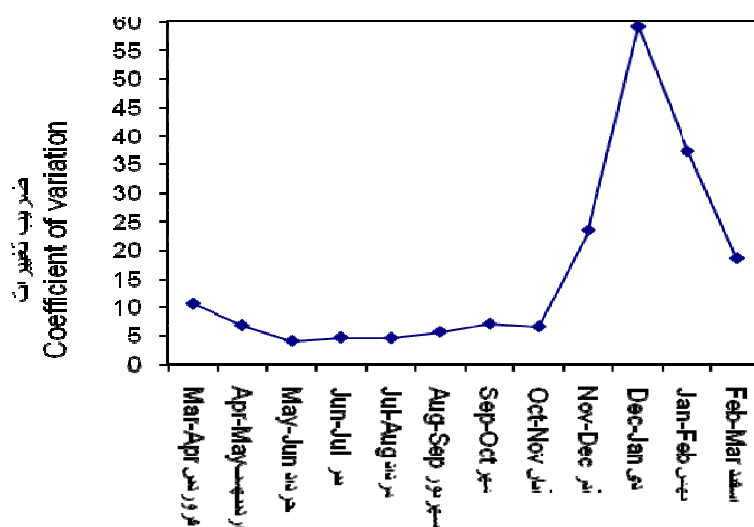
شکل ۱- ضریب تغییرات زمانی دما Fig. 1. Coefficient of temporal variation of temperature
