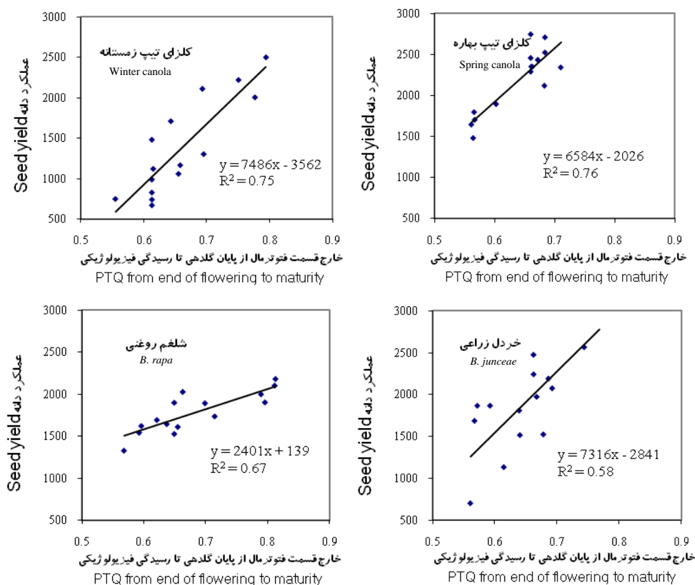
شکل ۳- رابطه بین عملکرد دانه (کیلوگرم در هکتار) و خارج قسمت فتوترمال (مگاژول بر متر مربع در روز در درجه سانتی‌گراد) طی دوره بین پایان گلدهی تا رسیدگی فیزیولوژیک
